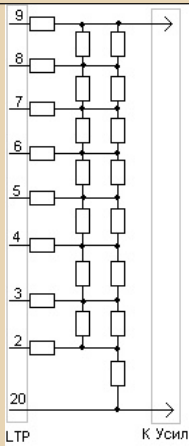
Рис.1 Схема Covox'a
